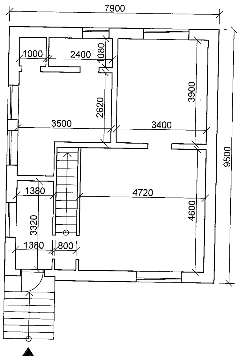
Põdorys 1.NP
