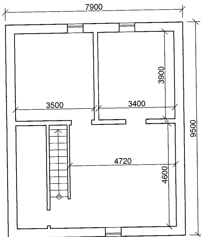
Pôdorys 1.PP
